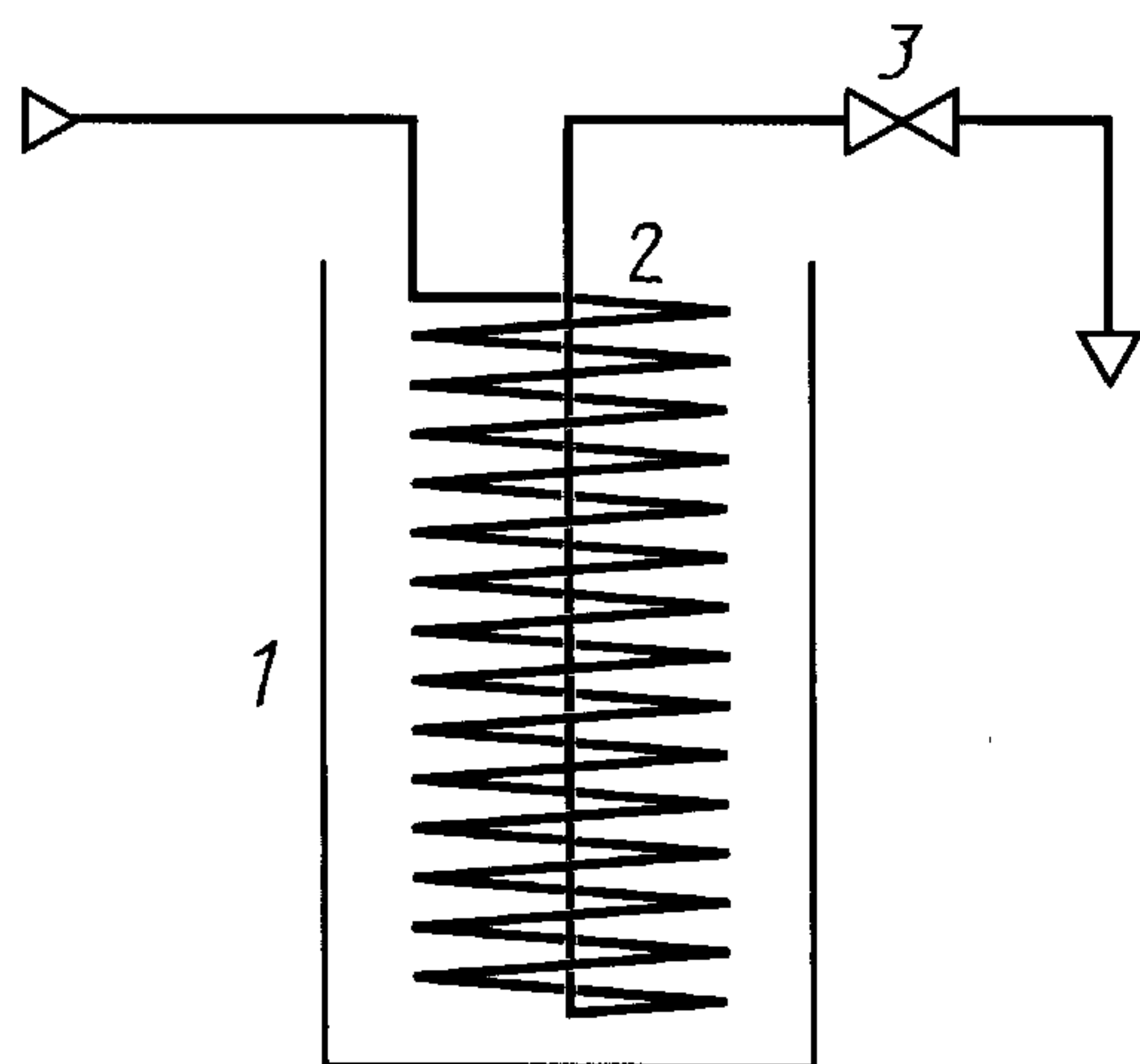
1 — сосуд для охлаждающей смеси; 2 — змеевик; 3 — игольчатый вентиль
